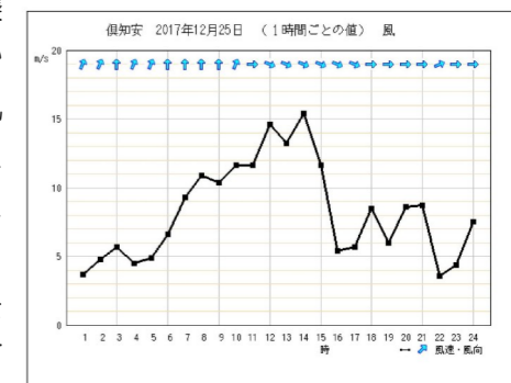
12月25日の風速推移（気象庁HPより）。昼過ぎに秒速15m以上の暴風が吹いたことがわかる。
